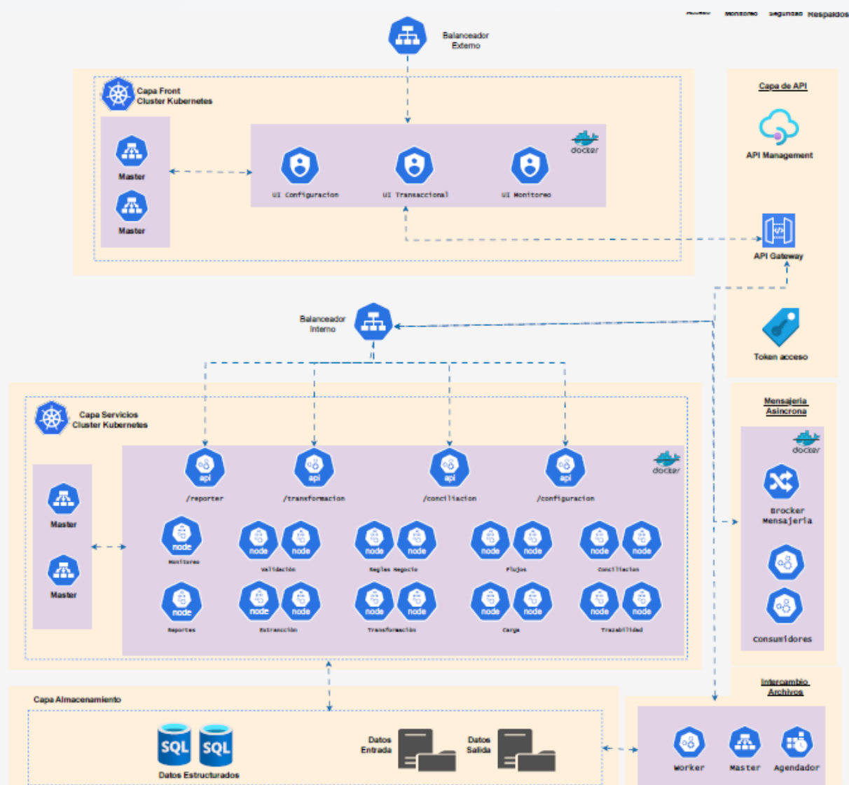
Figura 5. Arquitectura de la Suite modular - Capas Front, API, Servicios y Almacenamiento
